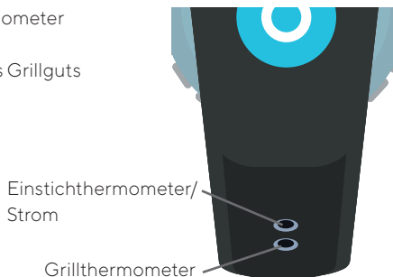
Abb. 9: Anschlussbuchsen
