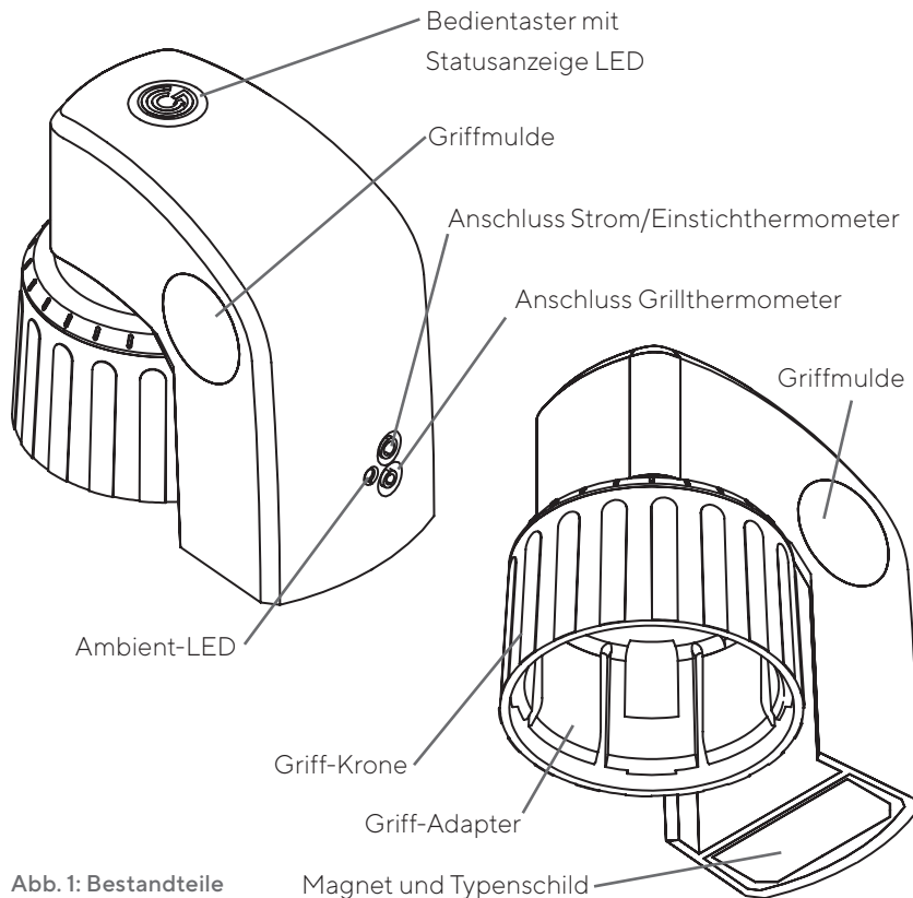
Abb. 1: Bestandteile
